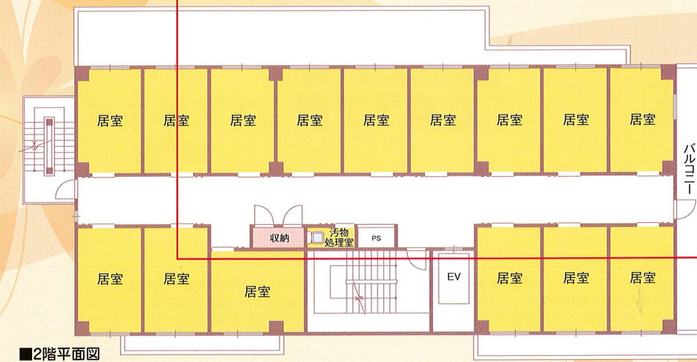
■2階平面図
