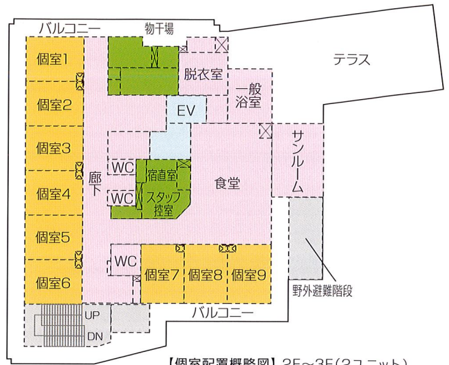
【個室配置概略図】2F~3F(2ユニット)
