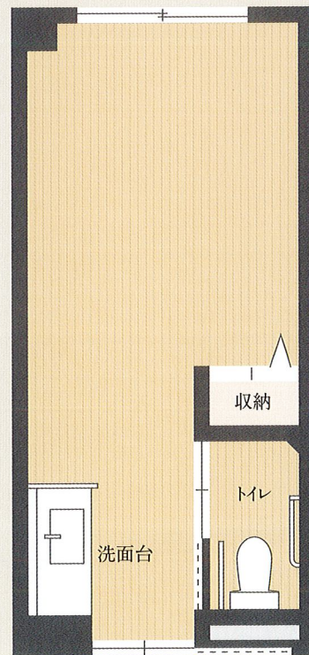
居室間取り一例
