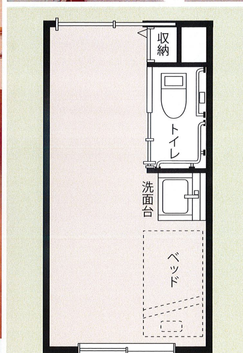
居室間取例
